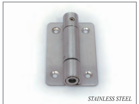
SSH7327 90mmL x 55mmW x 2mmT
